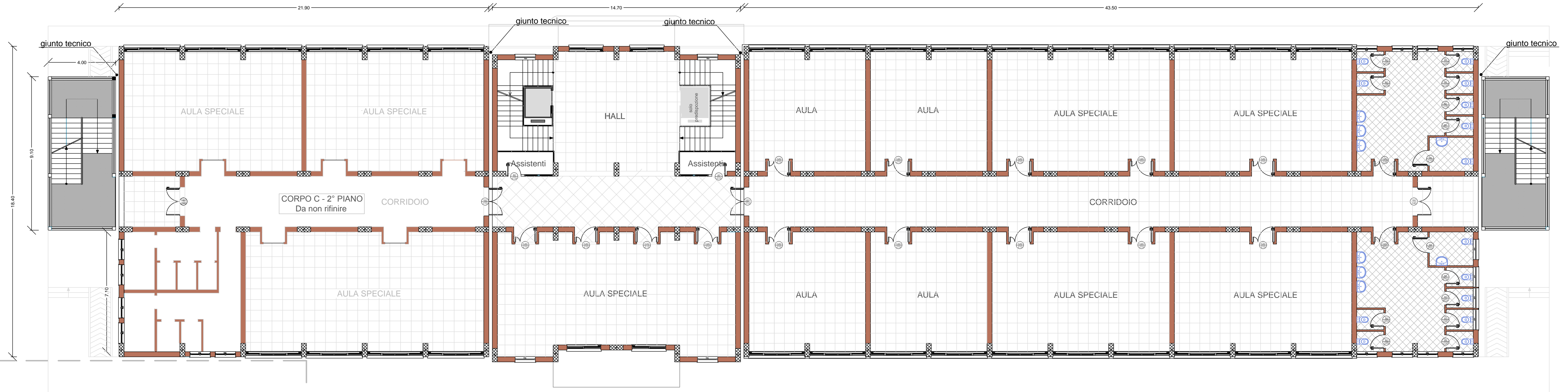
PIANTA SECONDO LIVELLO (Quota m 7.00) scala 1:100
